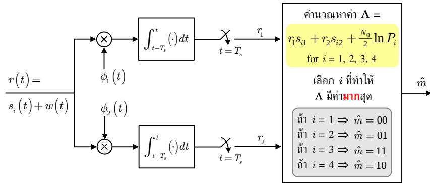
รูปที่ 7.19 โครงสร้างของวงจรภาครับสำหรับระบบ QPSK
